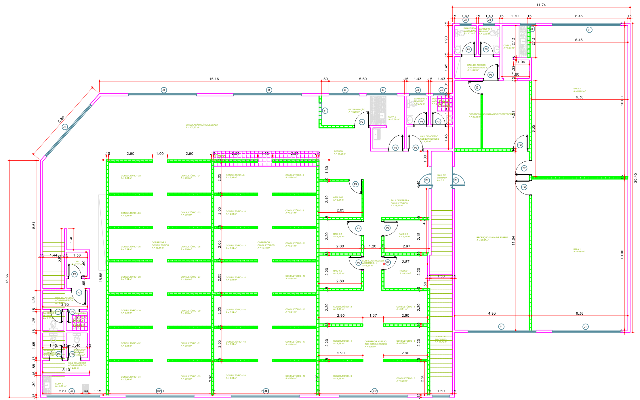
Planta Baixa Esc. 1:125
